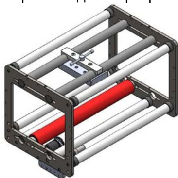
Рис. 58. Правильный вариант протяжки запечатываемого упаковочного материала
