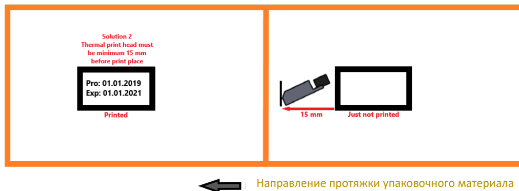
Рис. 47. Правильное положение остановки печатающей головки (Решение 2)
