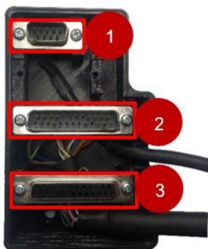
Рис. 34. Единая штепсельная вилка для кабелей принтера
