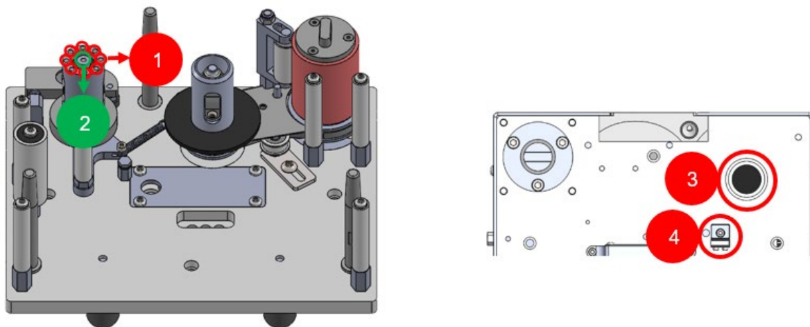
Рис. 59. Кассета (слева) и углубление для кассеты (справа)
