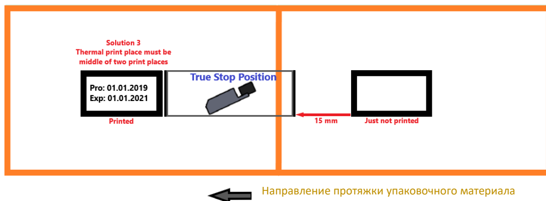
Рис. 48. Правильное положение остановки печатающей головки (Решение 3)
