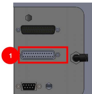
Рис. 57. Разъемы на принтере
