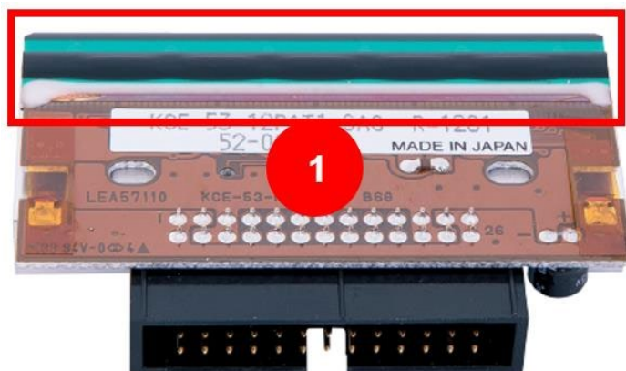
Рис. 60. Печатающая термоголовка Артикул: 200507-TPH
