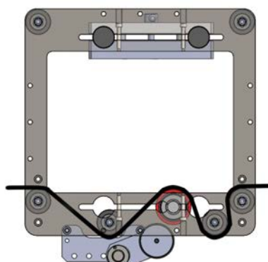
Рис. 58. Правильный вариант протяжки запечатываемого упаковочного материала
