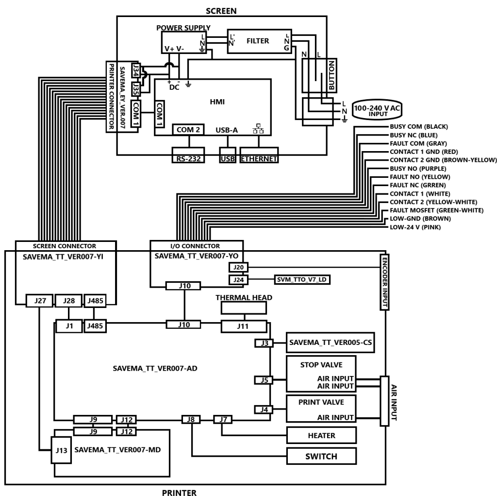
Рис. 24. Схема соединений плат и электронных компонентов
