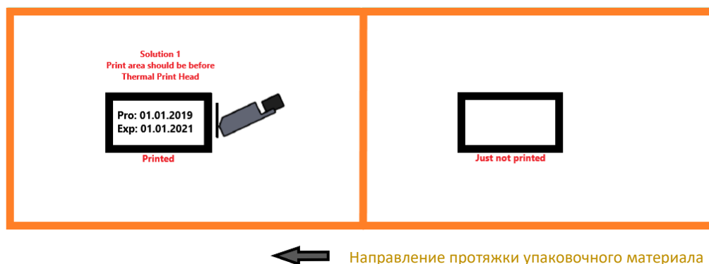
Рис. 46. Правильное положение остановки печатающей головки (Решение 1)
