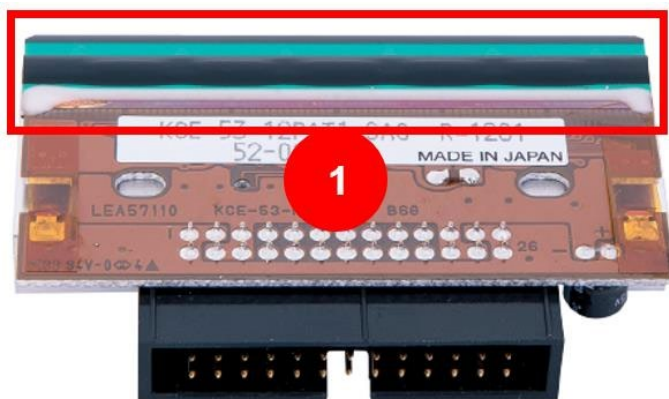
Рис. 62. Печатающая термоголовка Артикул: 200107-ТРН
