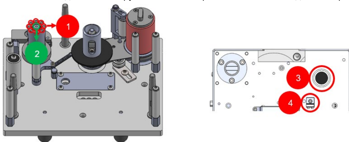
Рис. 61. Кассета (слева) и углубление для кассеты (справа)
