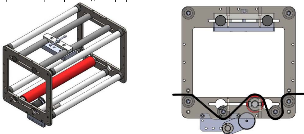
Рис. 60. Правильный вариант протяжки запечатываемого упаковочного материала
