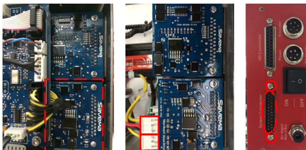
Рис. 53. Замена платы связи с блоком управления
