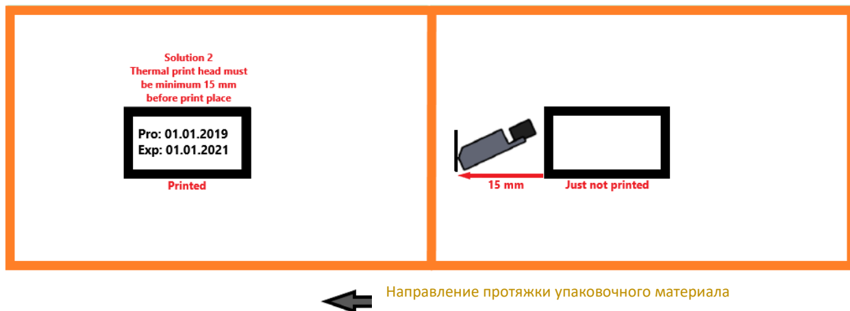
Рис. 47. Правильное положение остановки печатающей головки (Решение 2)
