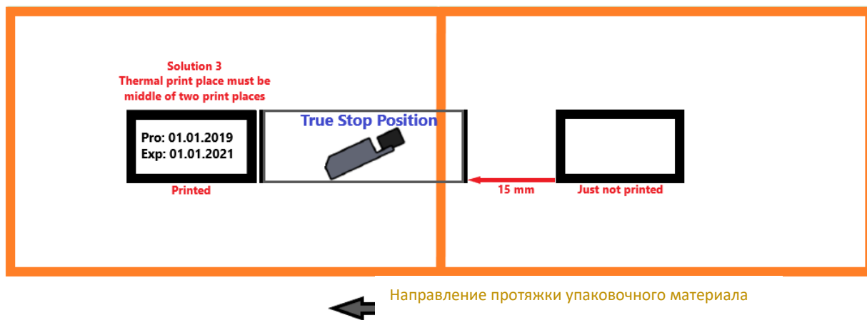
Рис. 48. Правильное положение остановки печатающей головки (Решение 3)
