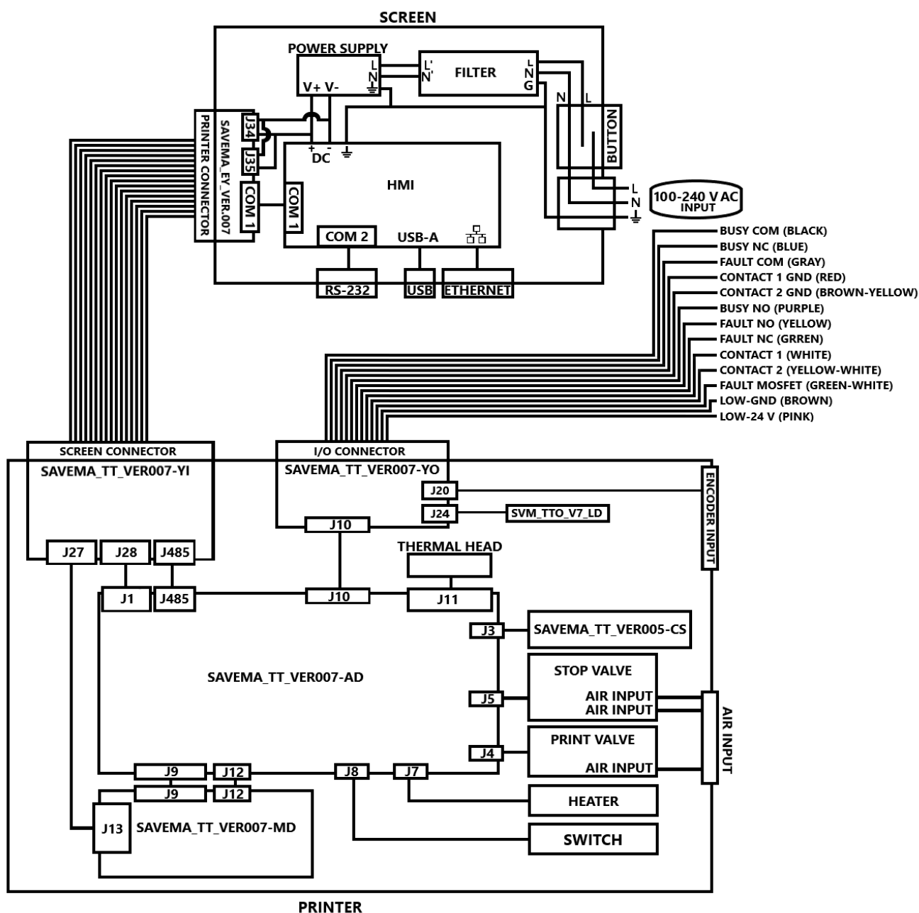
Рис. 24. Схема соединений плат и электронных компонентов
