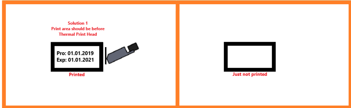
Рис. 46. Правильное положение остановки печатающей головки (Решение 1)
