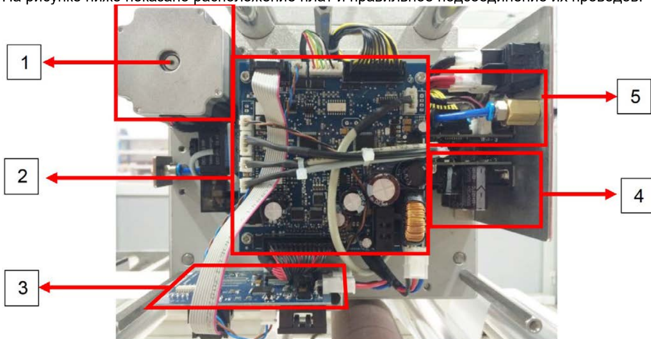
Рис. 55. Расположение электронных плат в принтере
