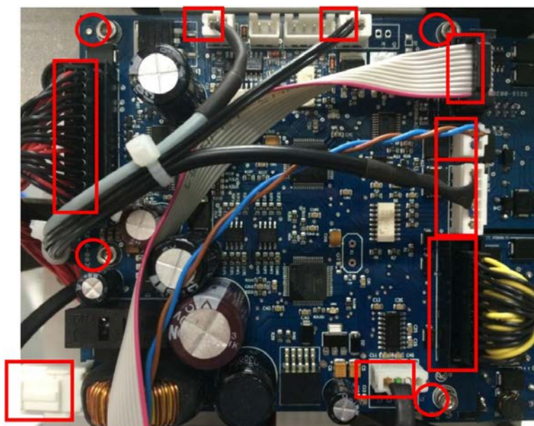
Рис. 51. Замена материнской платы
