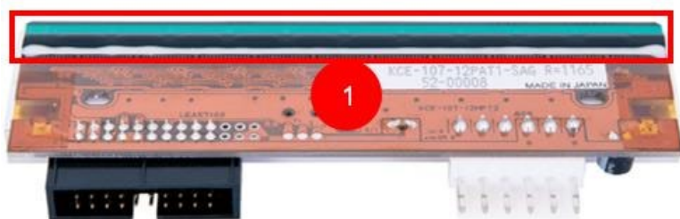
Рис. 62. Печатающая термоголовка Артикул: 200207-ТРН
