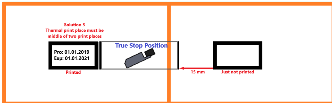
Рис. 48. Правильное положение остановки печатающей головки (Решение 3)
