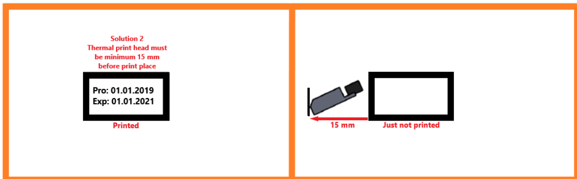
Рис. 47. Правильное положение остановки печатающей головки (Решение 2)
