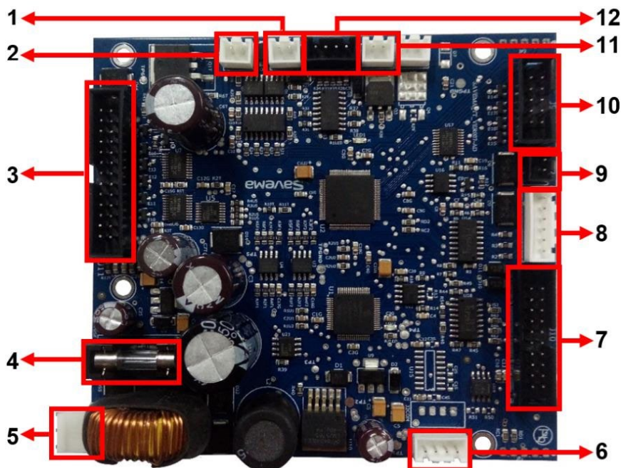
Рис. 56. Расположение разъемов на материнской плате
