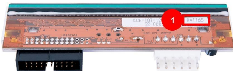
Рис. 20. Печатающая термоголовка
