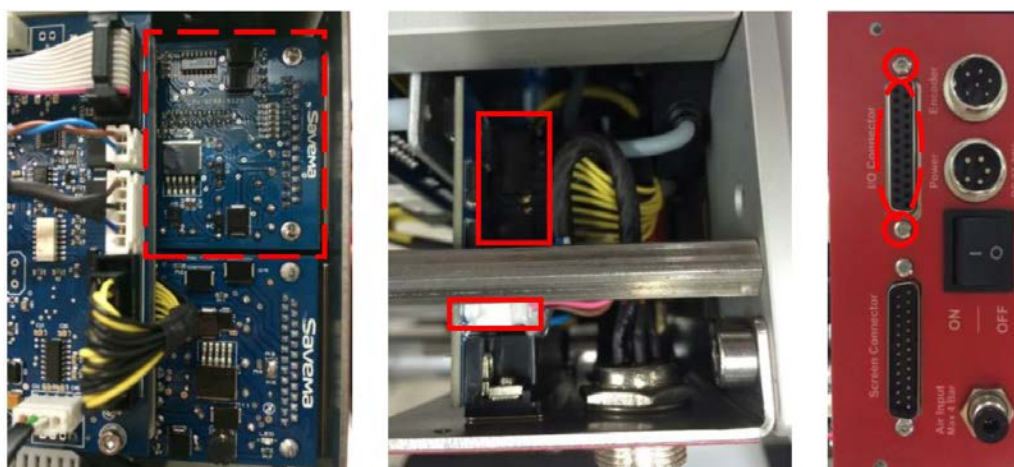
Рис. 54. Замена сигнальной платы
