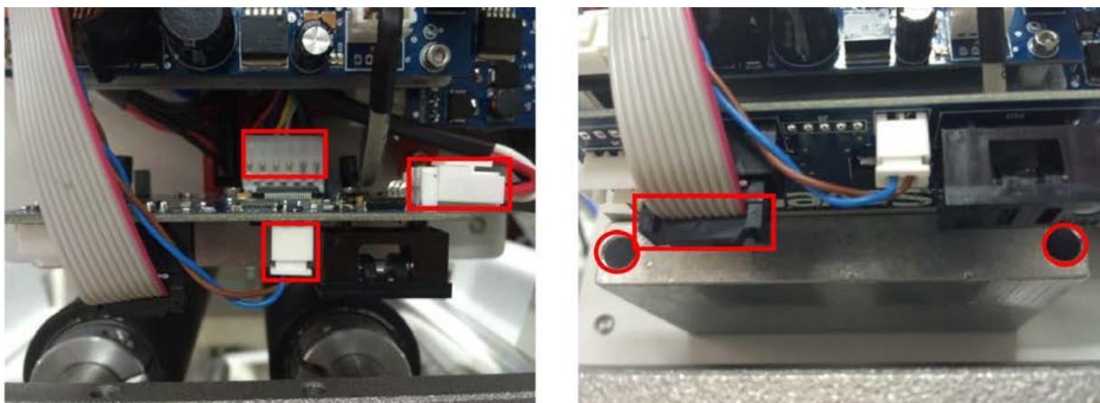
Рис. 52. Замена микросхемы-драйвера двигателей
