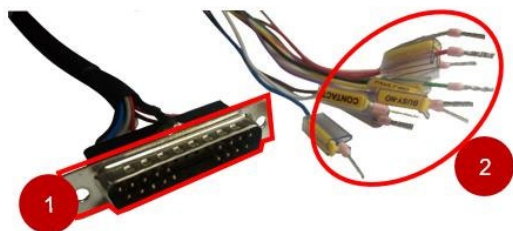
Рис. 37. Сигнальный кабель Артикул: C-CNTV7
