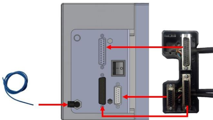
Рис. 39. Панель принтера и единая штепсельная вилка с разъемами следующих кабелей: сигнального кабеля, кабеля связи с блоком управления и кабеля для подключения блока питания.
