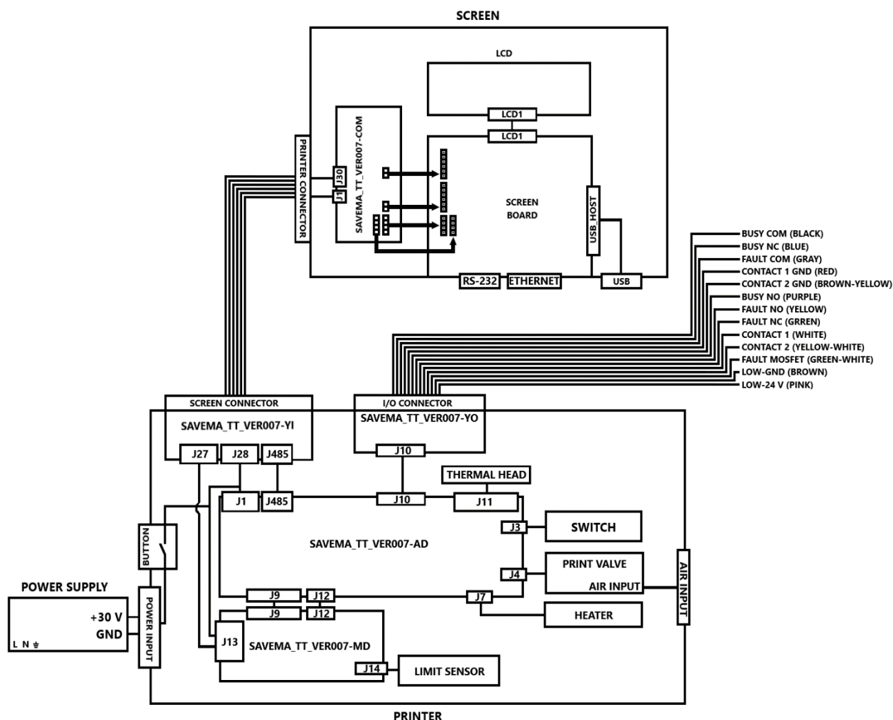
Рис. 22. Схема соединений плат и электронных компонентов
