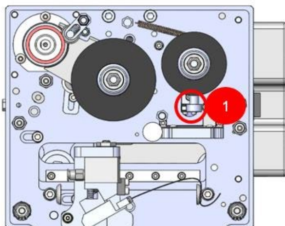
Рис. 51. Система обнаружения обрыва риббона
