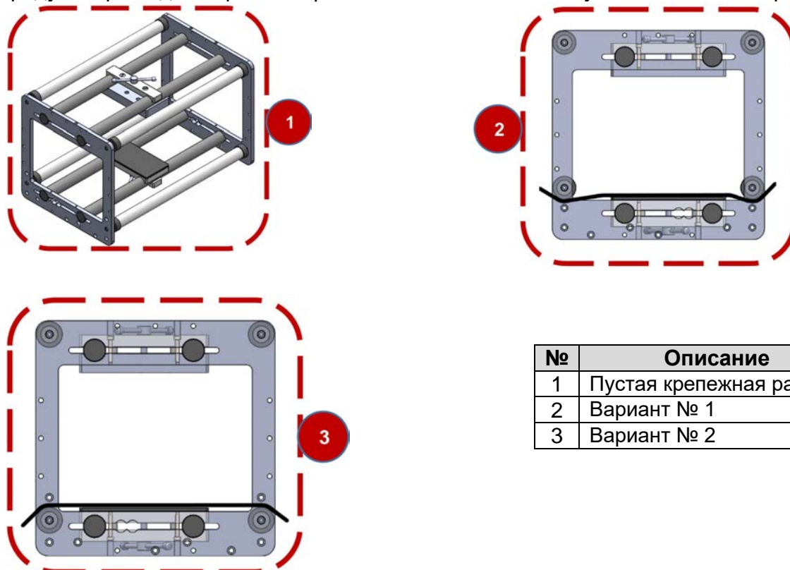
Рис. 50. Правильные варианты протяжки запечатываемого упаковочного материала
