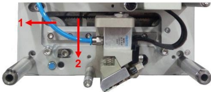
Рис. 21. Изображение ведущего вала и ходового ремня
