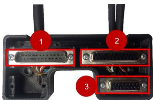
Рис. 33. Единая штепсельная вилка для кабелей принтера
