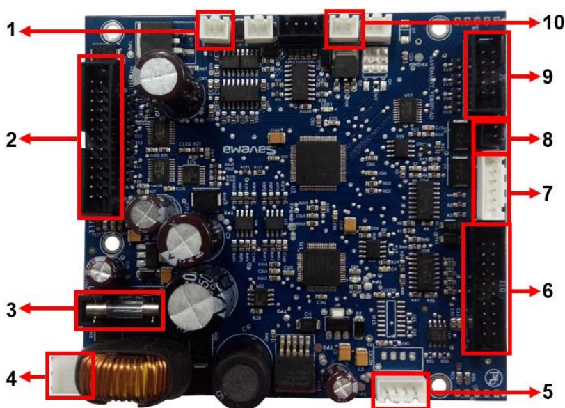
Рис. 44. Расположение разъемов на материнской плате
