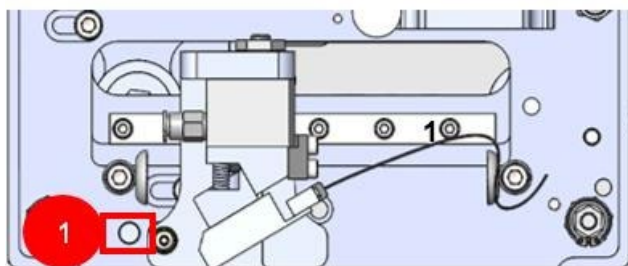
Рис. 54. Датчик предельного перемещения по горизонтали
