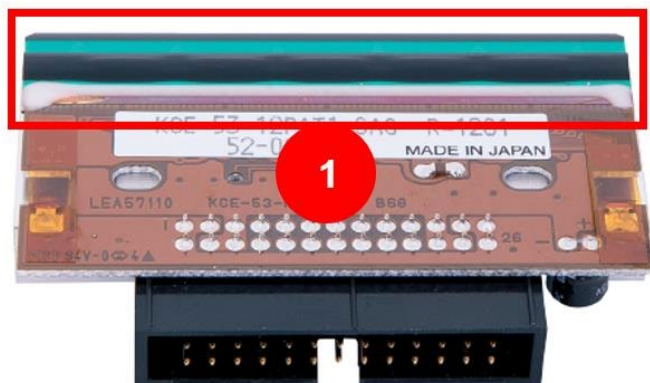
Рис. 52. Печатающая термоголовка Артикул: 200117-TPH
