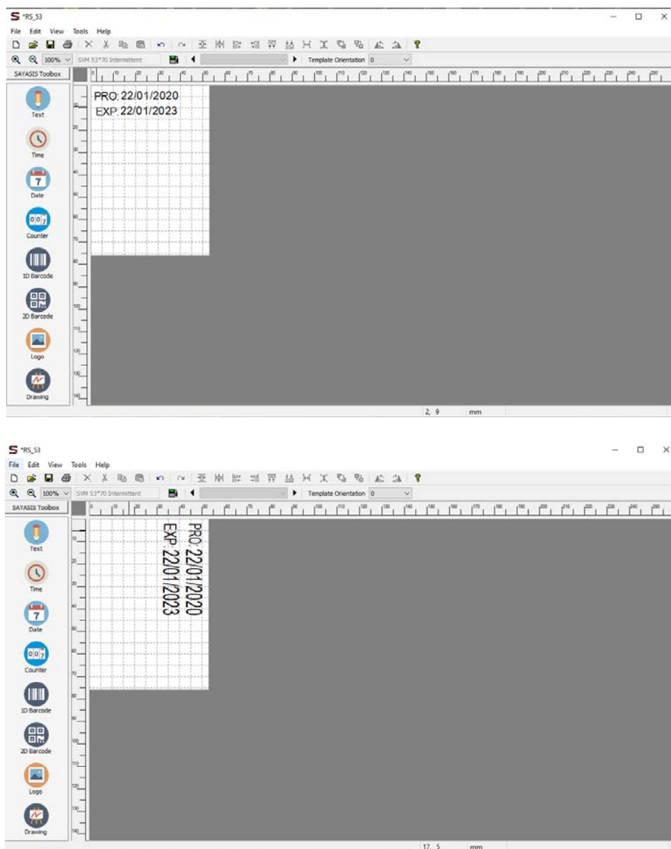
Рис. 7. Шаблон маркировки, пригодный для использования функции экономии риббона по вертикали. Вариант №1 (вверху) и вариант №2 (внизу).
