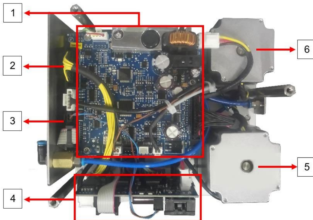
Рис. 43. Расположение электронных плат в принтере
