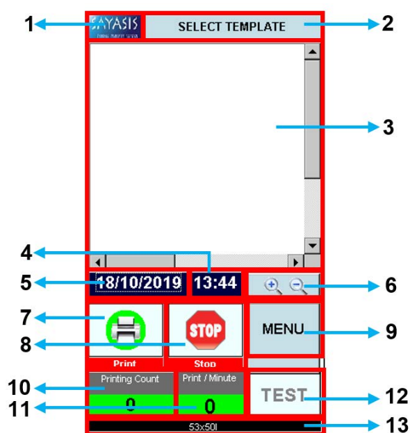
Рис. 1. Главное меню
