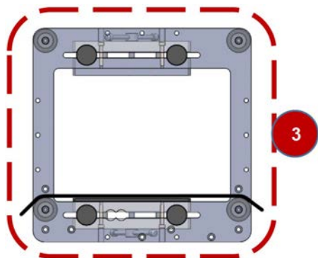
Рис. 47. Правильные варианты протяжки запечатываемого упаковочного материала
