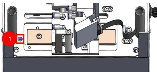
Рис. 51. Датчик предельного перемещения по горизонтали
