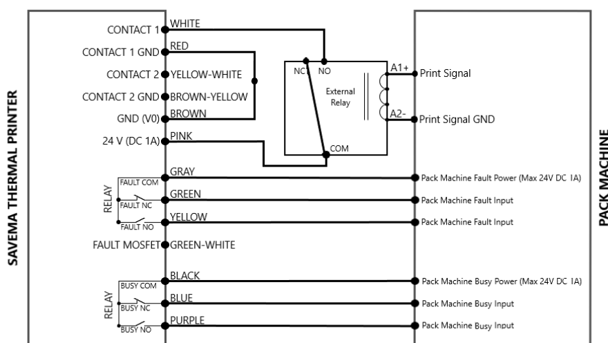
Рис. 24. Схема подключения реле PNP (на рисунке реле обозначено как External Relay)
