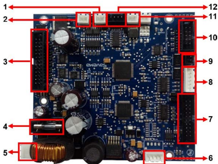
Рис. 41. Расположение разъемов на материнской плате
