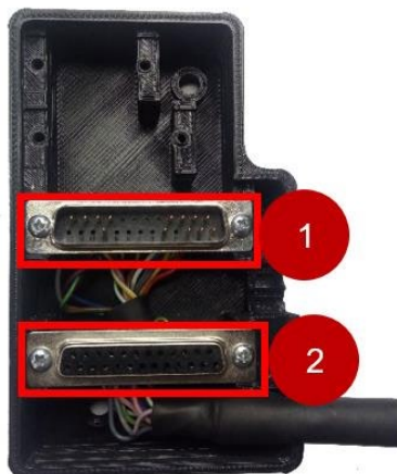
Рис. 29. Единая штепсельная вилка для кабелей принтера
