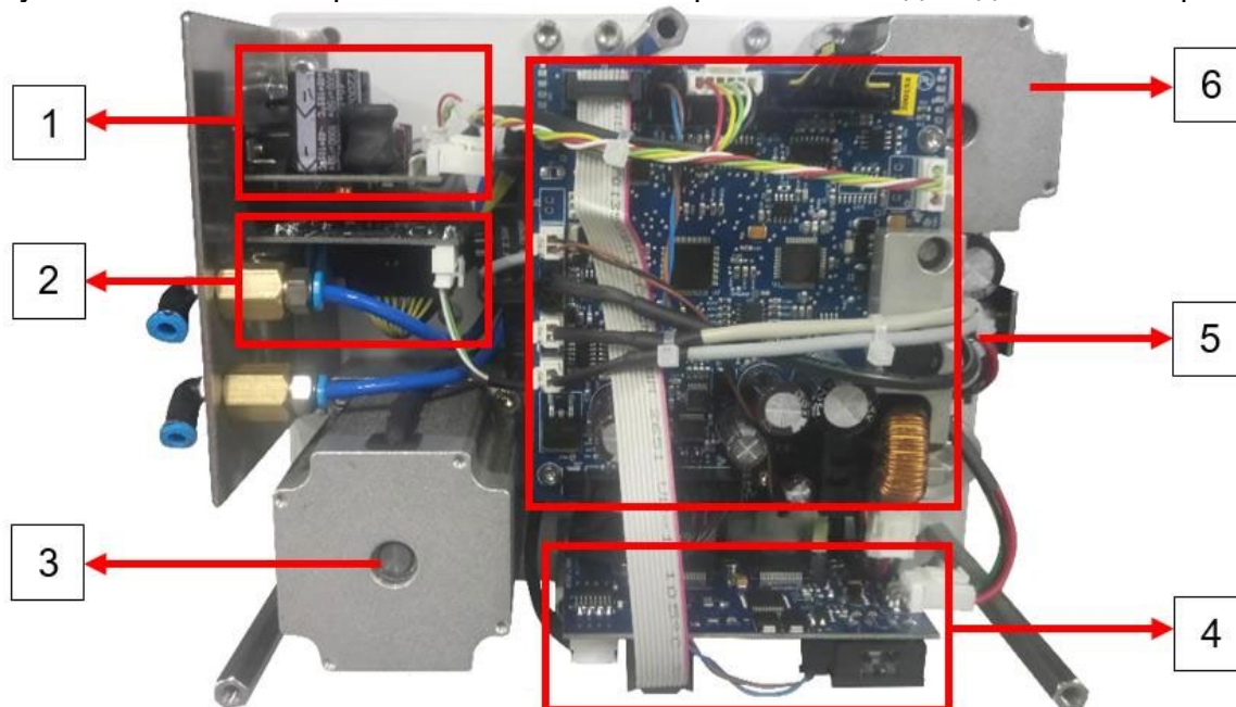
Рис. 40. Расположение электронных плат в принтере
