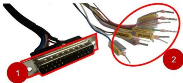
Рис. 34. Сигнальный кабель Артикул: С-CNTV7
