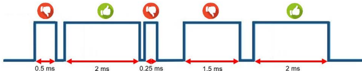
Рис. 15. Пример, когда минимальная длительность импульса внешнего сигнала печати установлена на 2 мс
